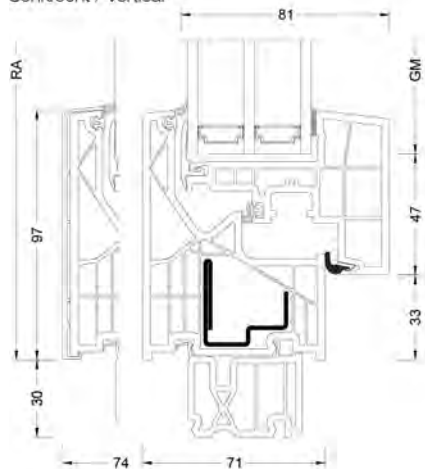
Senkrecht / Vertical
